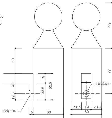
支柱連結部詳細図 1/2
