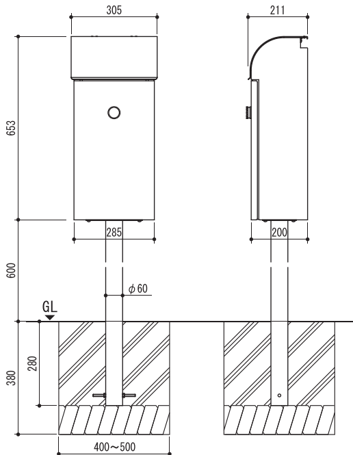
■寸法図
