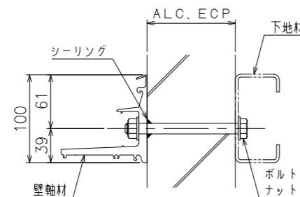
ALC、ECP下地に取付ける場合
