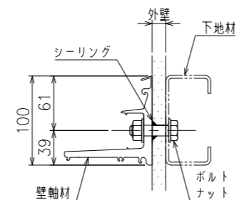
鉄骨下地に取付ける場合
