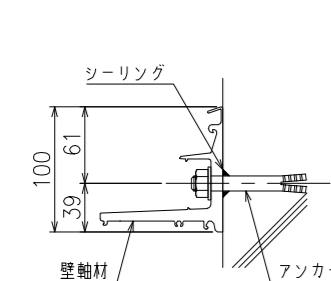
コンクリート下地に取付ける場合
