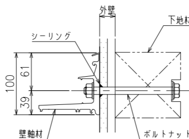
木下地に取付ける場合
