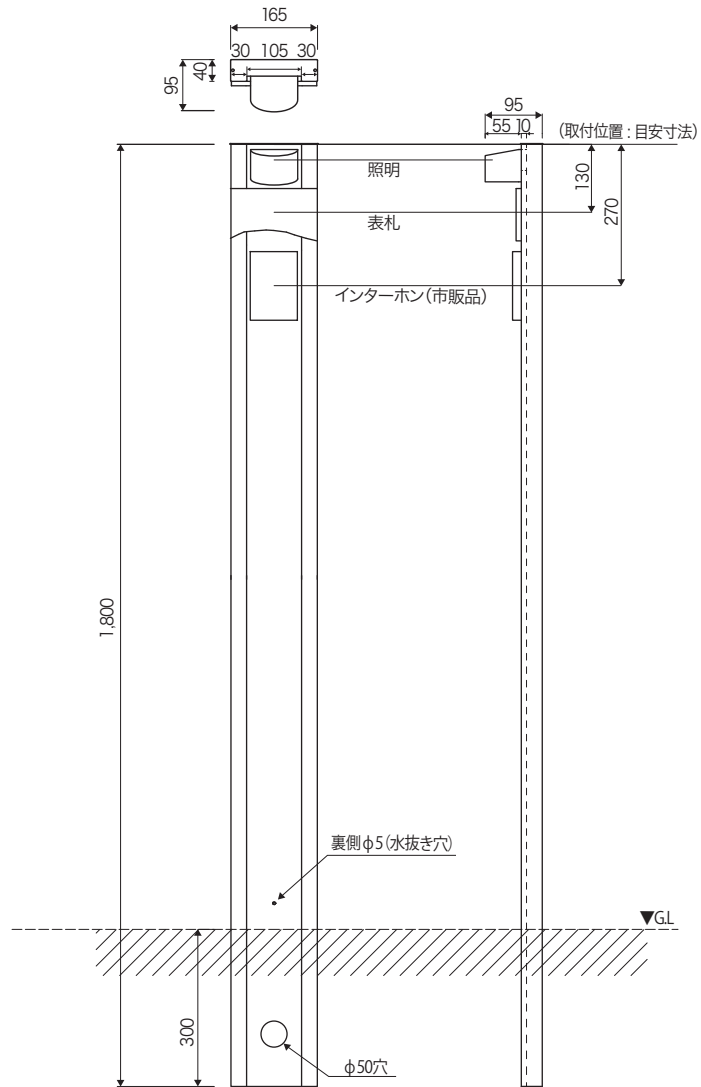
〈本体正面図〉
