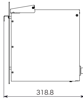
〈本体側面図〉
