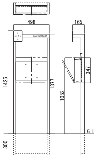
●Wタイプ (IP+LED) 仕様
