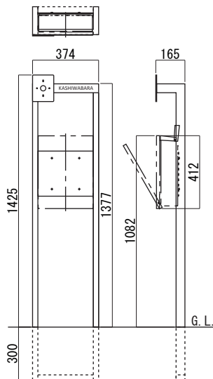
●Sタイプ (IP+LED) 仕様
