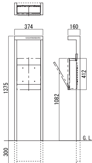
●Sタイプ (LED) 仕様
