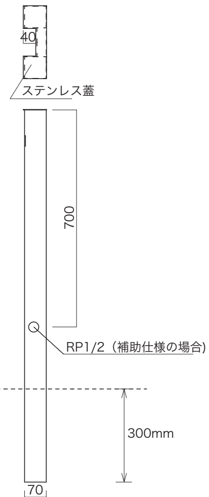
〈側面図〉
