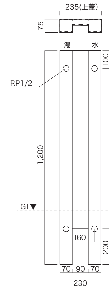
〈上面図〉
