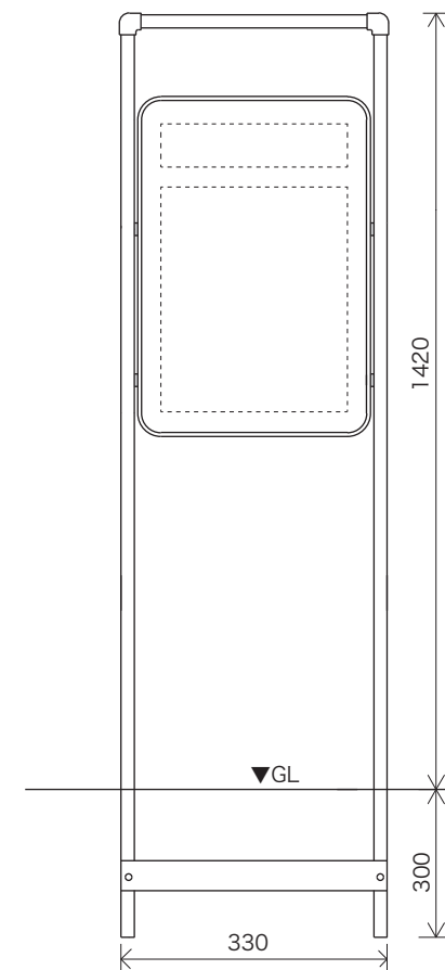
〈専用スタンド正面図〉
