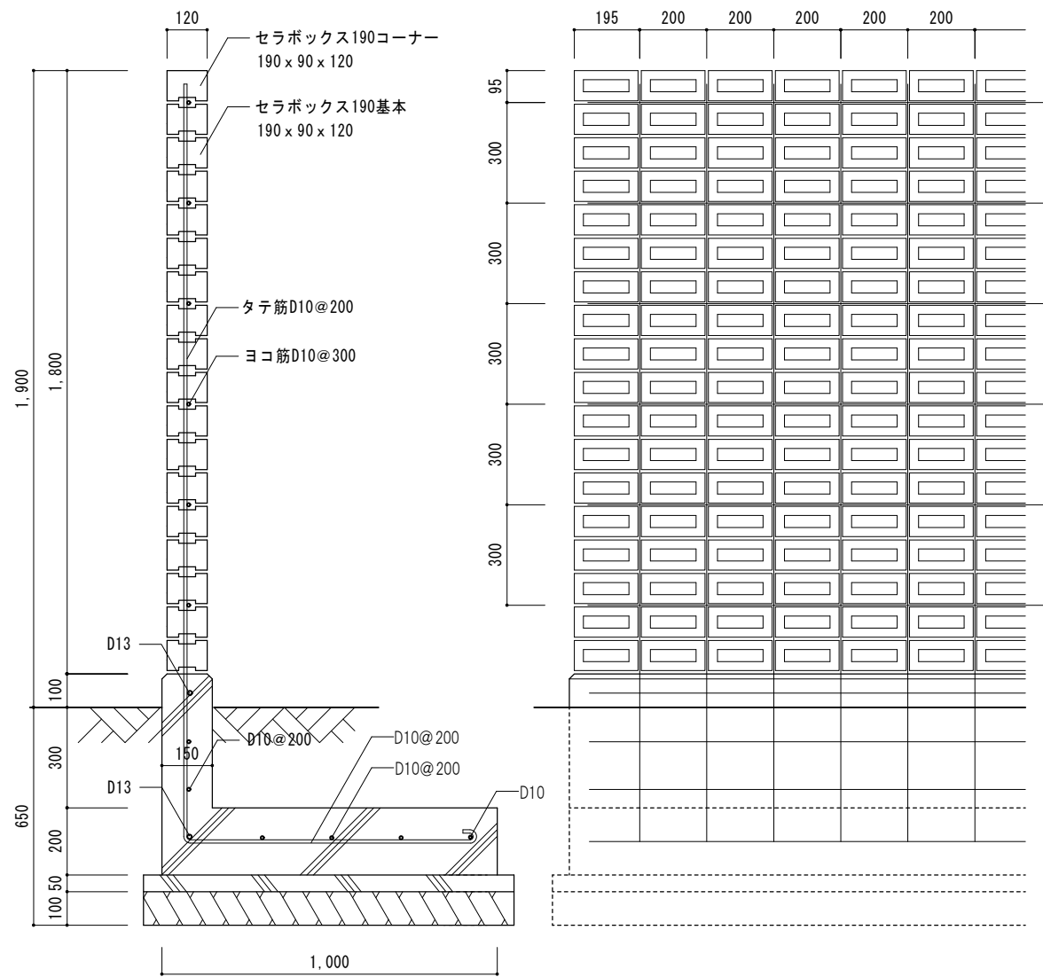
断面図 S=1:20
