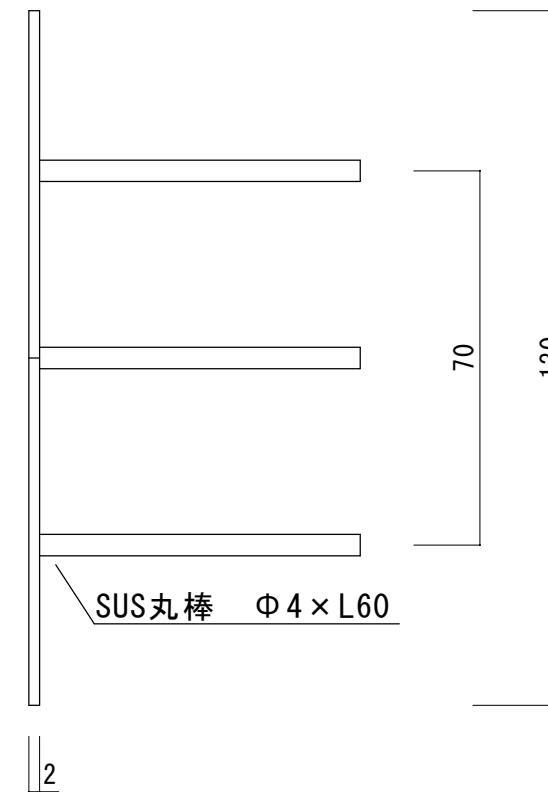
側面図
