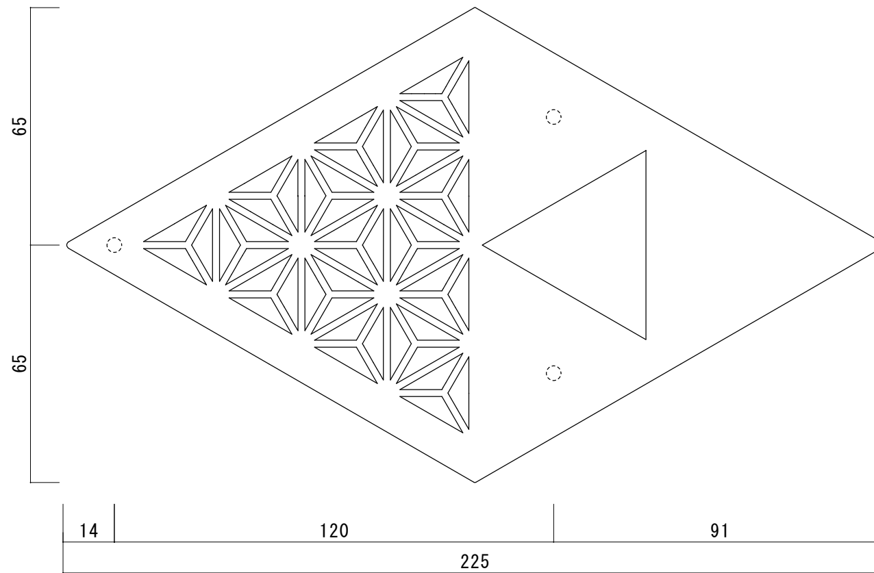
背面図
