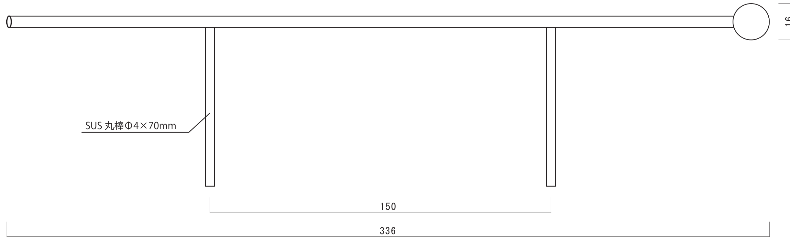
側面図
