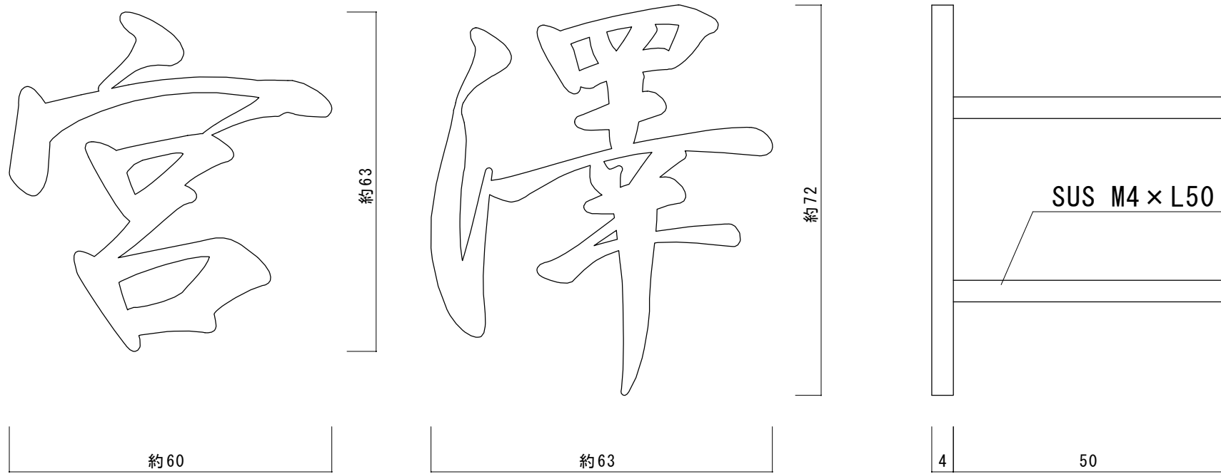
側面図
