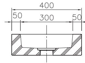
B-B断面図
