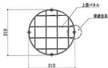
A 断面図 S=1:10
