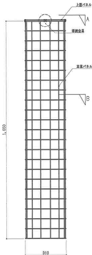
正面図 S=1:10
