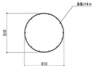
B 断面図 S=1:10
