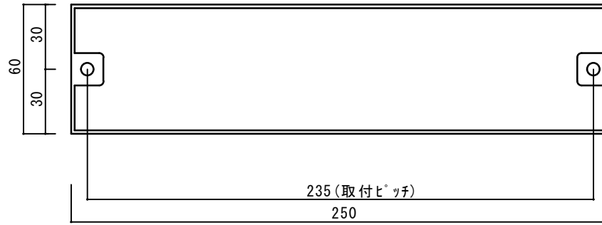
背面図
