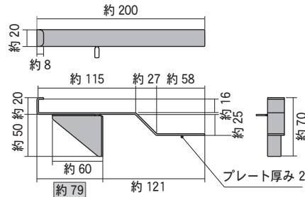
ワイドタイプ受け金具
