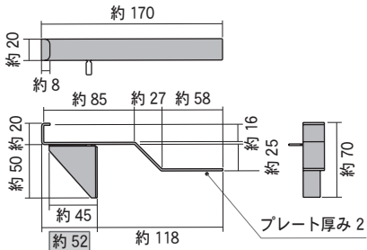
スリムタイプ受け金具
