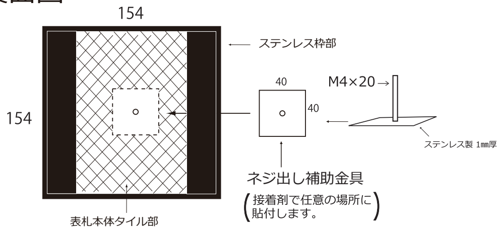
裏面図
