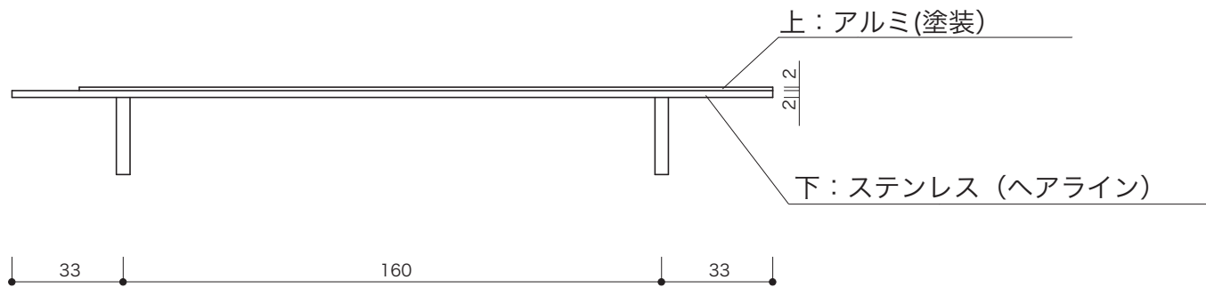
〈側面図〉
