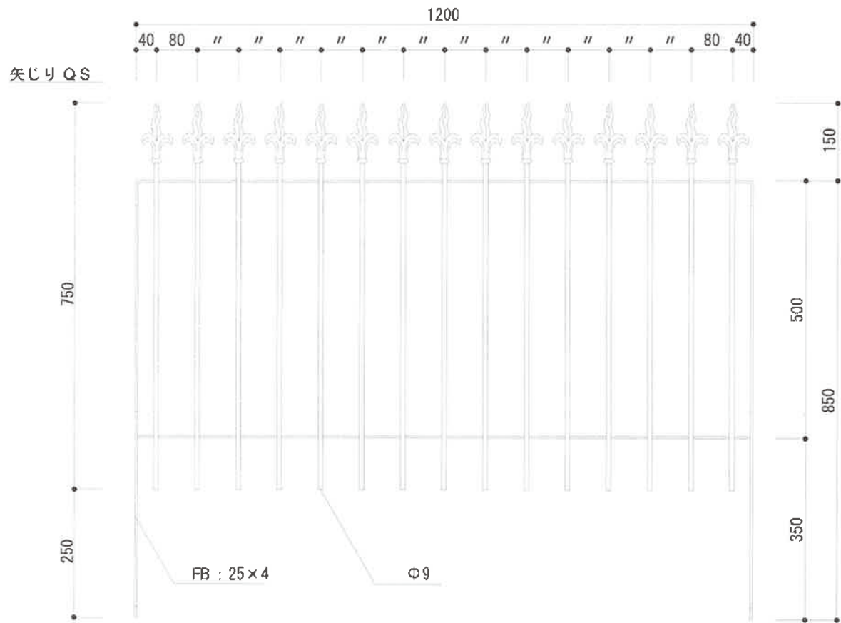
立面図 S=1/10
