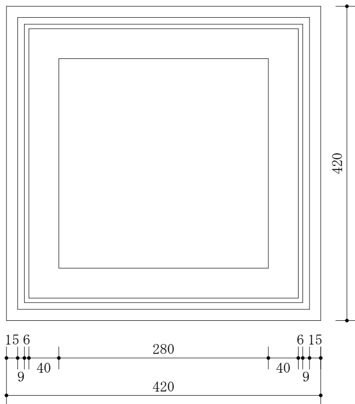
◆ 底面図
