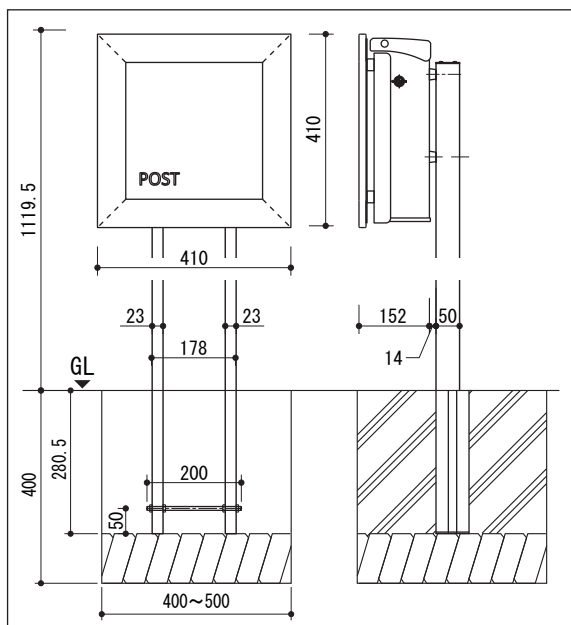
■寸法図
