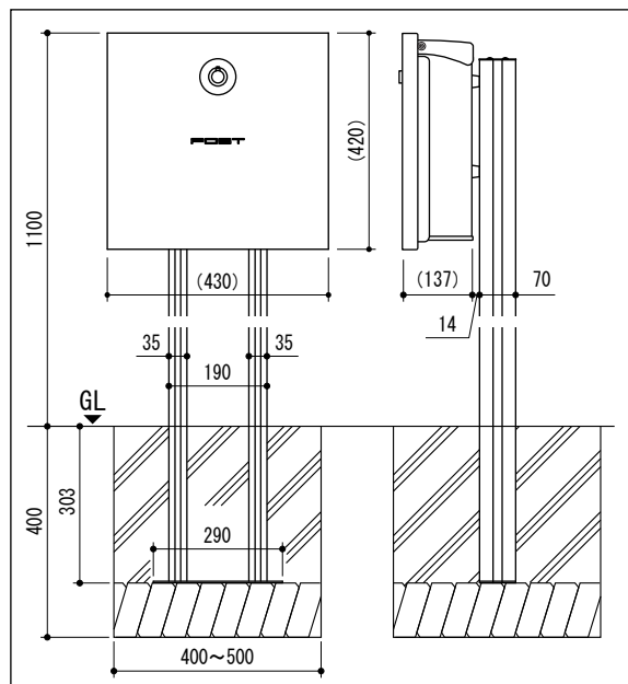
■ 寸法図
