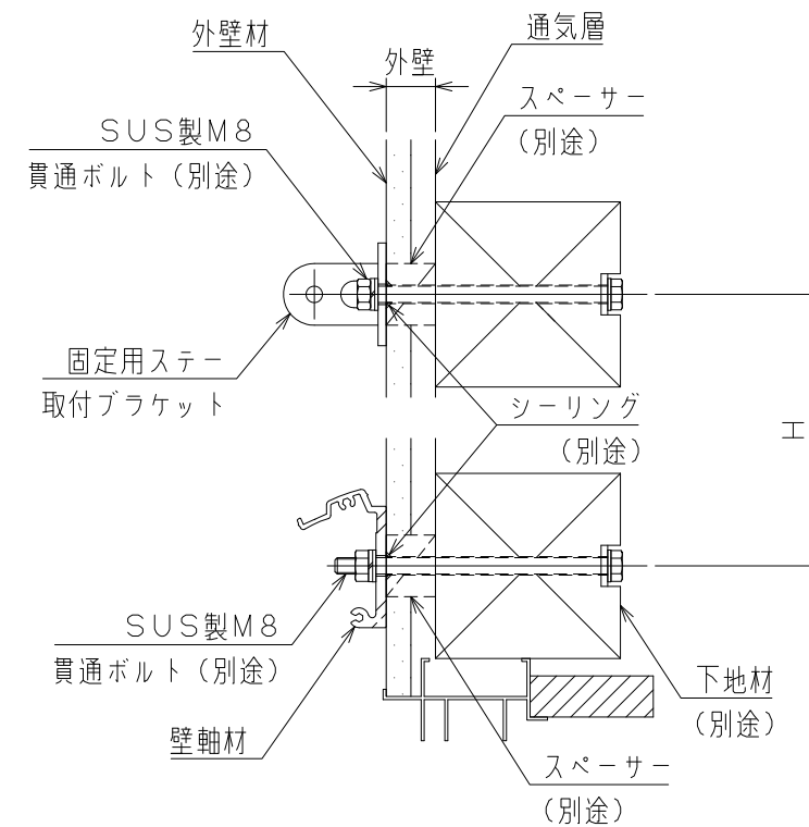
木下地に取付ける場合
