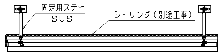
正面図
