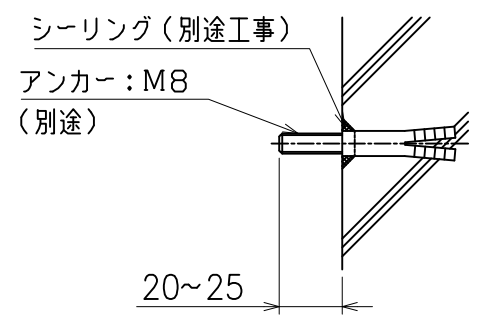
アンカー取付要領
