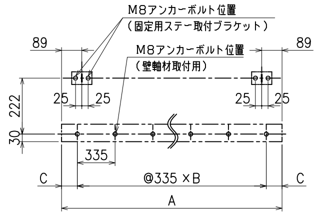
アンカー図
