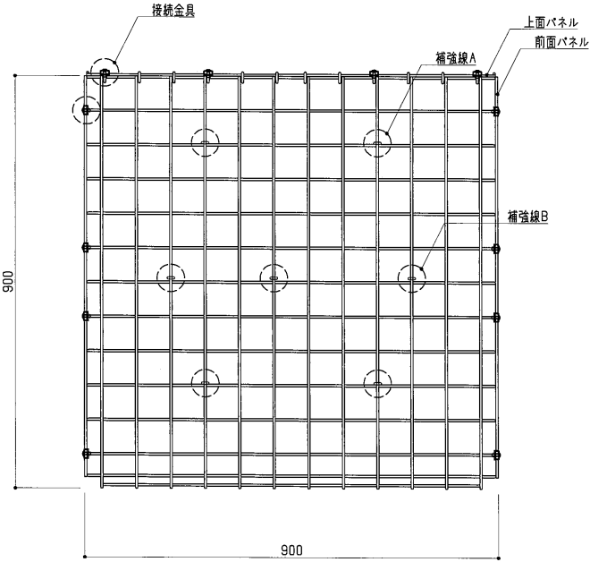
正面図 S=1:10
