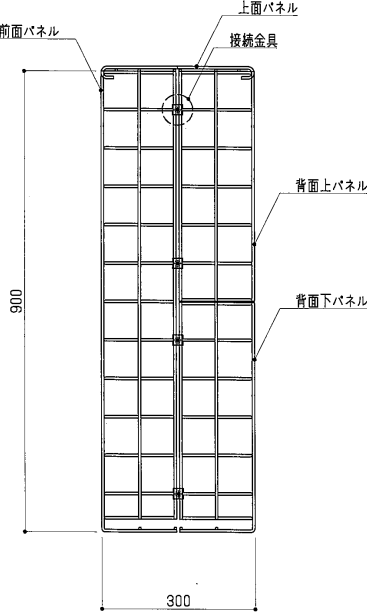
側面図 S=1:10
