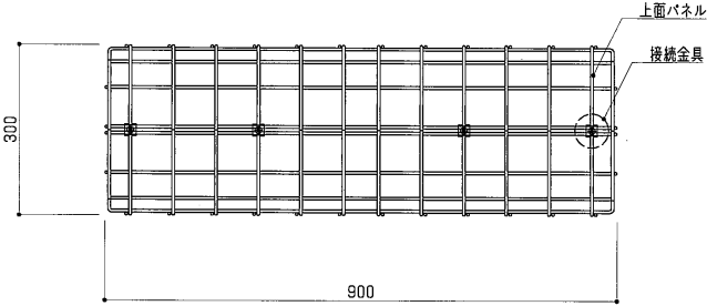
平面図 S=1:10
