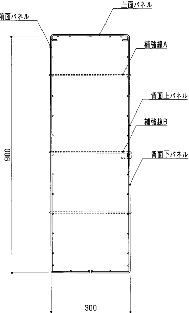
断面図 S=1:10
