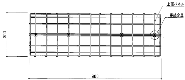
平面図 S=1:10
