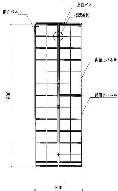
側面図 S=1:10
