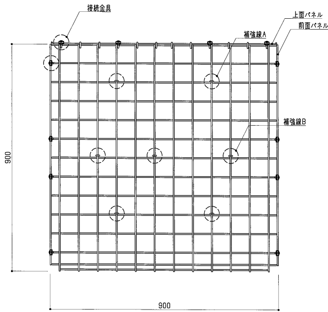
正面図 S=1:10
