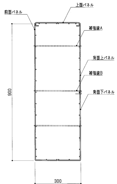
断面図 S=1:10
