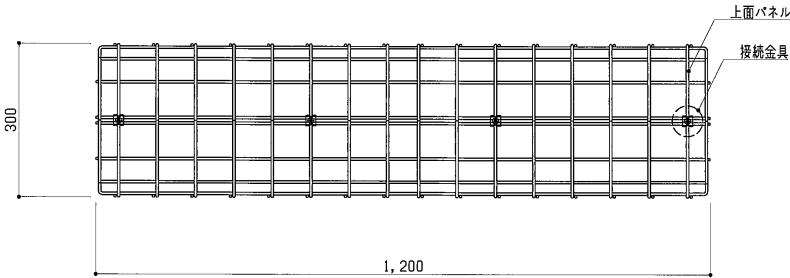
平面図 S=1:10
