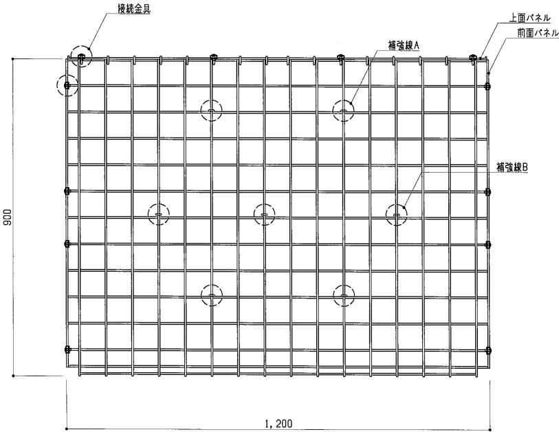
正面図 S=1:10
