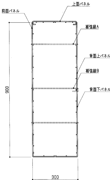
断面図 S=1:10
