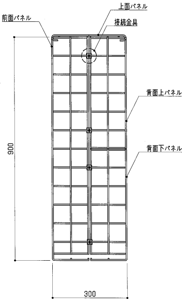
側面図 S=1:10
