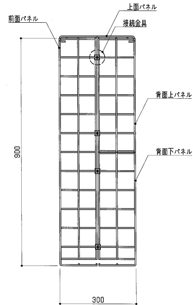
側面図 S=1:10
