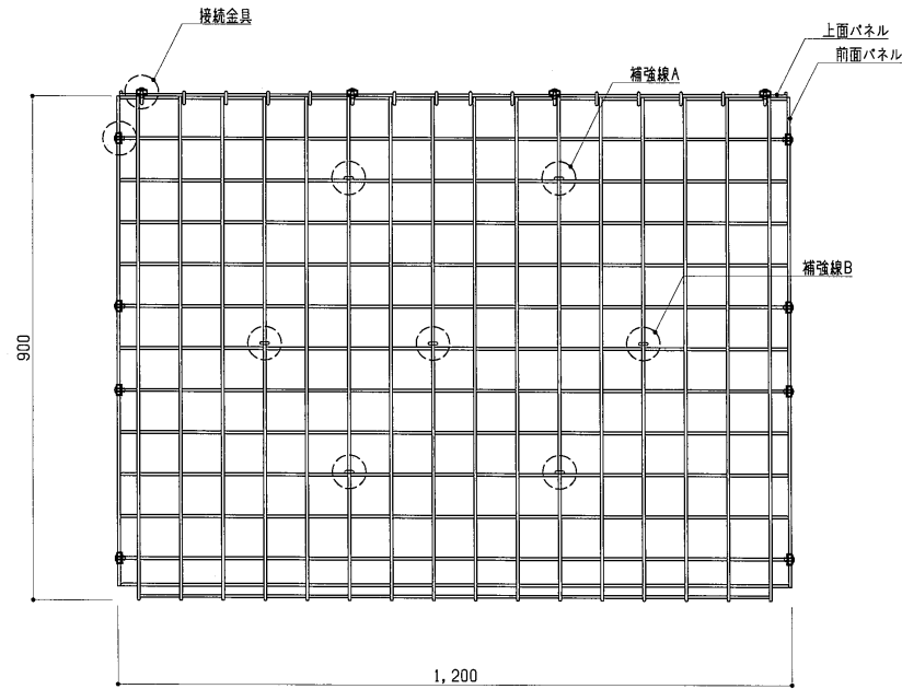
正面図 S=1:10
