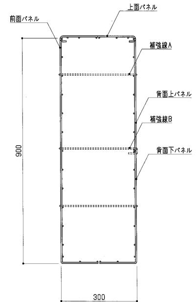
断面図 S=1:10
