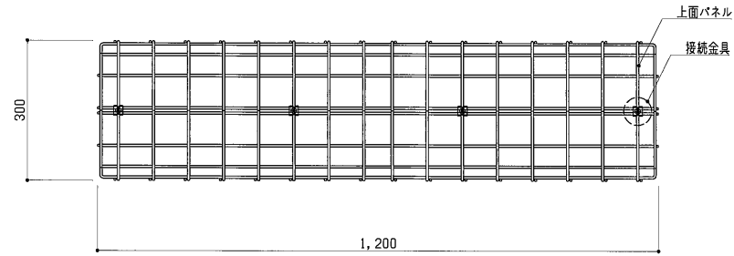
平面図 S=1:10
