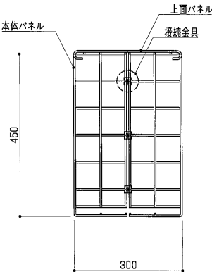
側面図 S=1:10
