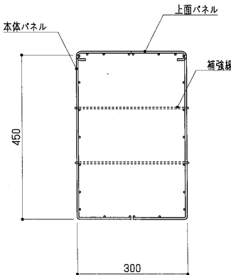
断面図 S=1:10
