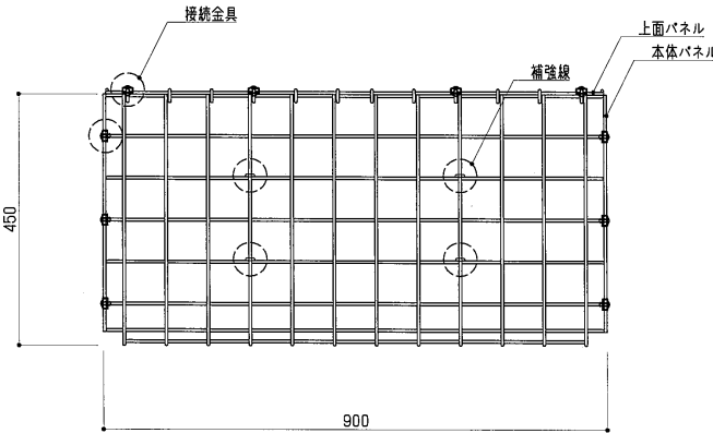
正面図 S=1:10
