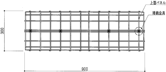
平面図 S=1:10
