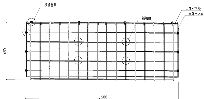
正面図 S = 1 : 10
