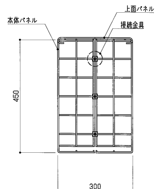
側面図 S = 1 : 10
