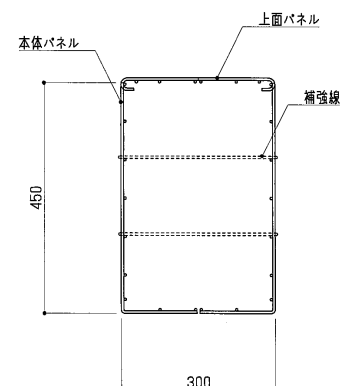
断面図 S = 1 : 10
