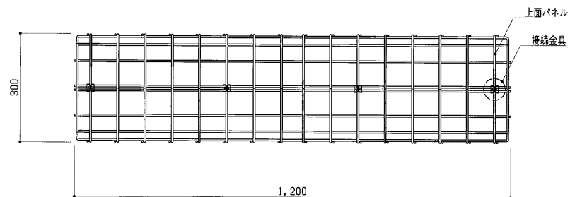
平面図 S = 1 : 10
