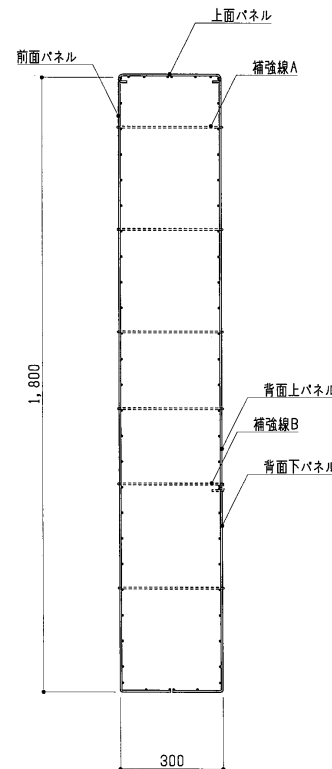
断面図 S=1:15
