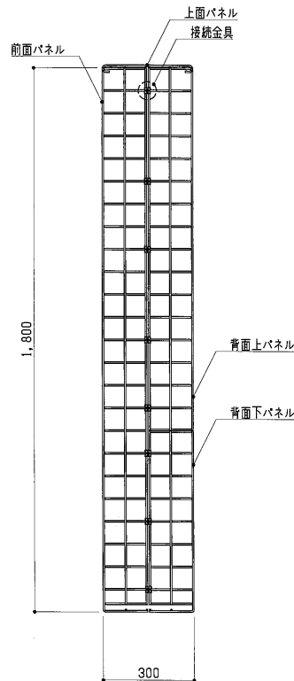
側面図 S=1:15
