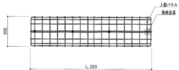
平面図 S=1:15
