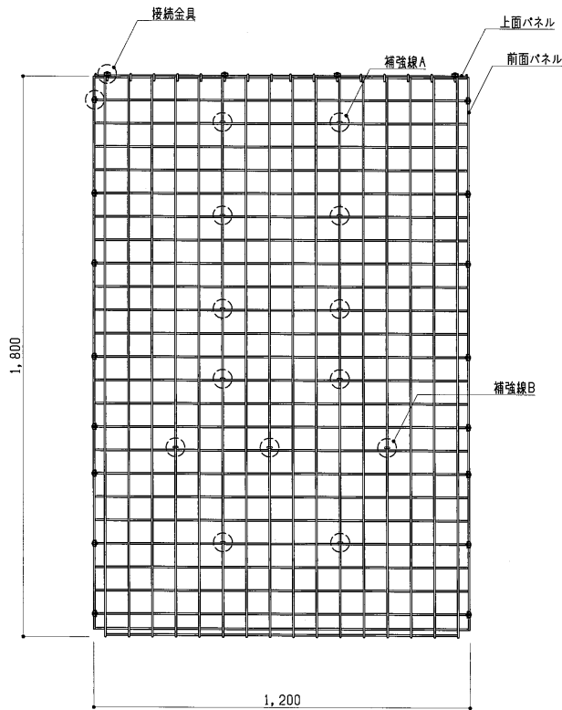
正面図 S=1:15
