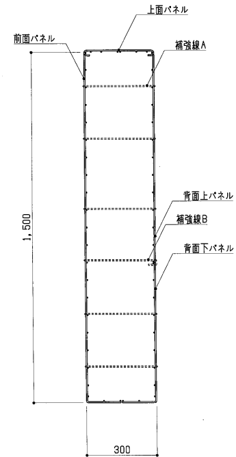
断面図 S = 1 : 15
