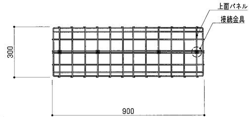
平面図 S = 1 : 15
