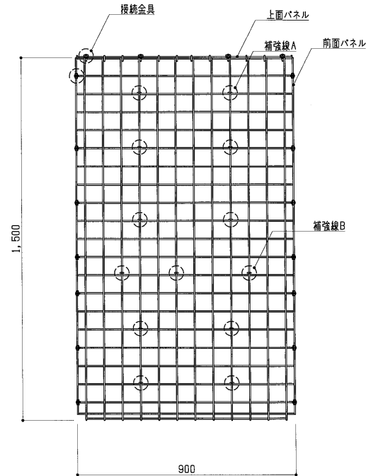
正面図 S = 1 : 15
