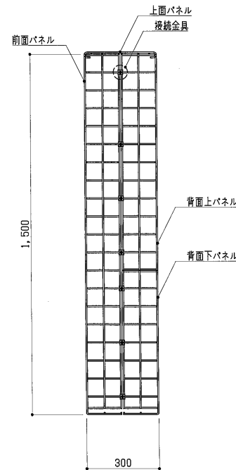
側面図 S = 1 : 15
