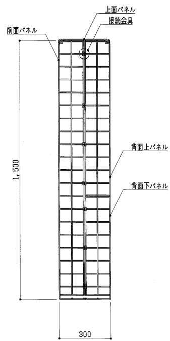
側面図 S=1:15
