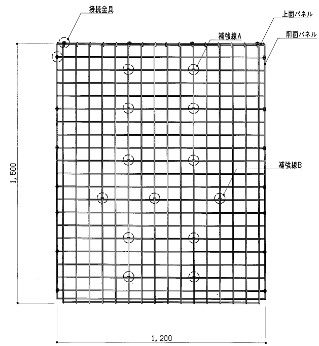
正面図 S=1:15
