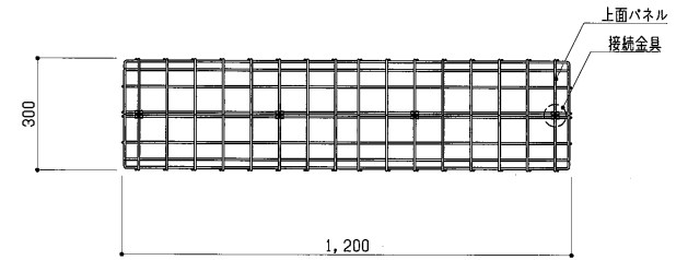
平面図 S=1:15
