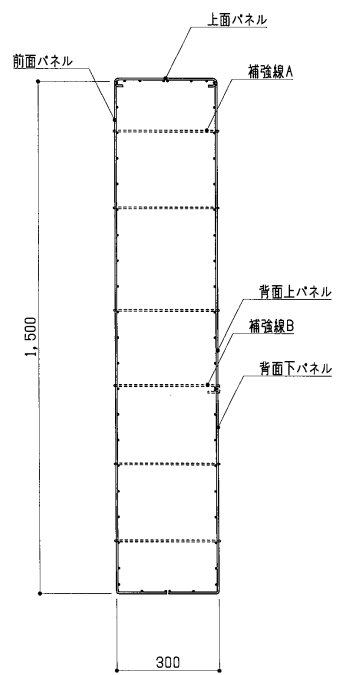
断面図 S=1:15
