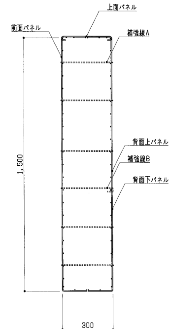
断面図 S=1:15
