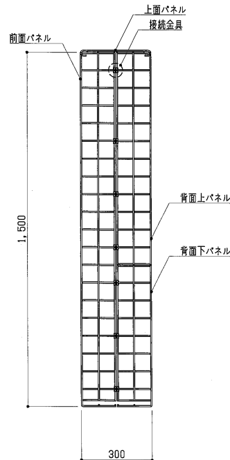
側面図 S=1:15
