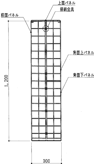
側面図 S=1:15
