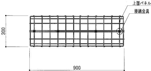
平面図 S=1:15
