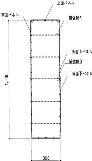
断面図 S=1:15
