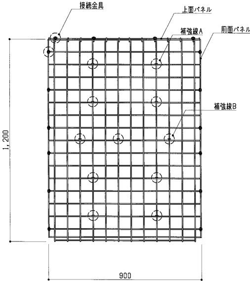
正面図 S=1:15
