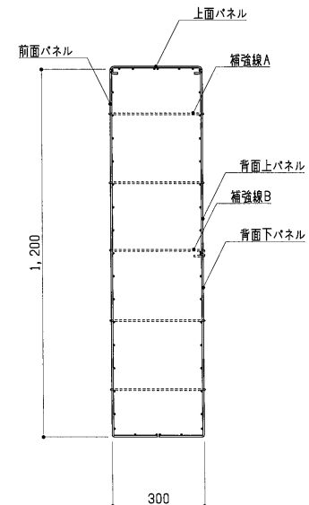
断面図 S=1:15
