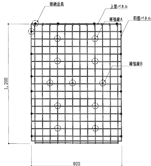
正面図 S=1:15
