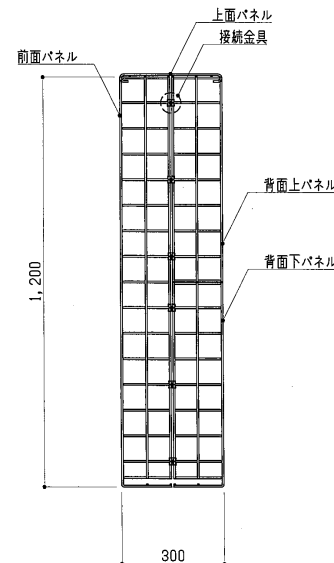
側面図 S=1:15
