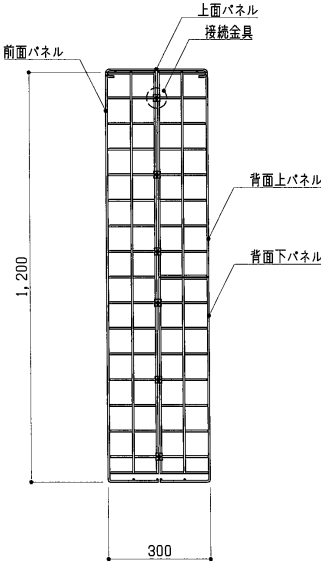
側面図 S=1:15
