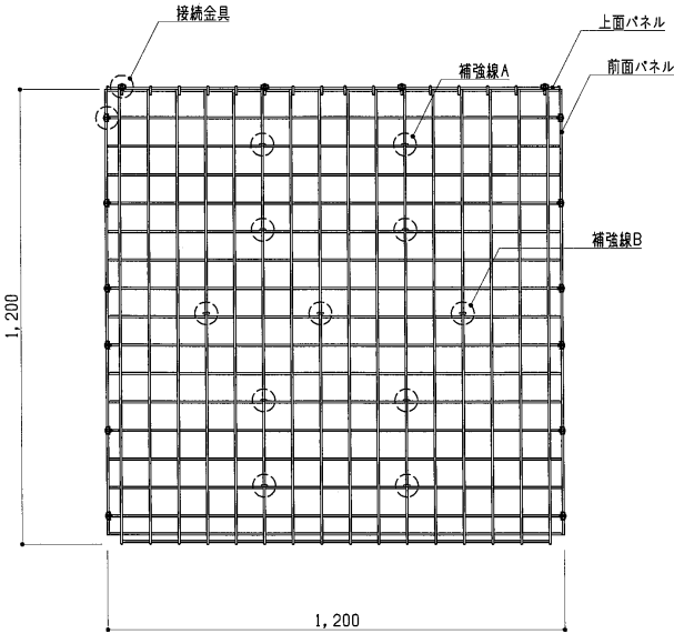
正面図 S=1:15
