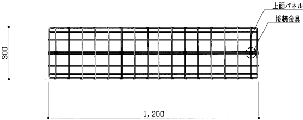
平面図 S=1:15
