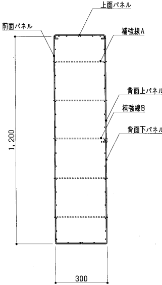
断面図 S=1:15
