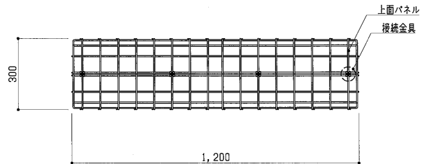
平面図 S = 1 : 15
