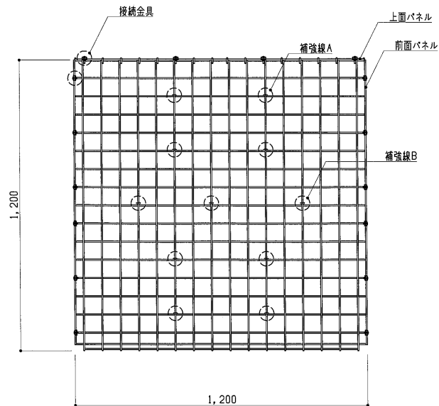
正面図 S = 1 : 15
