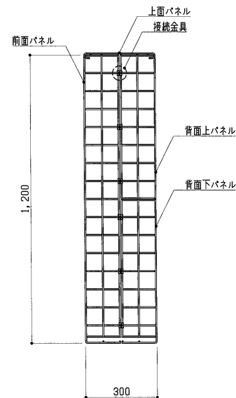
側面図 S = 1 : 15
