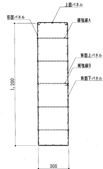
断面図 S = 1 : 15
