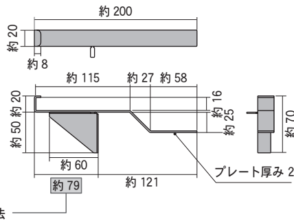
ワイドタイプ受け金具
