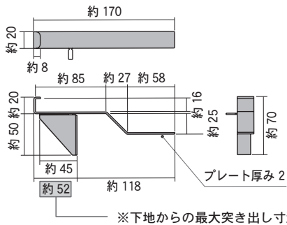
スリムタイプ受け金具
