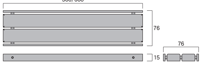
ワイドタイプ本体
