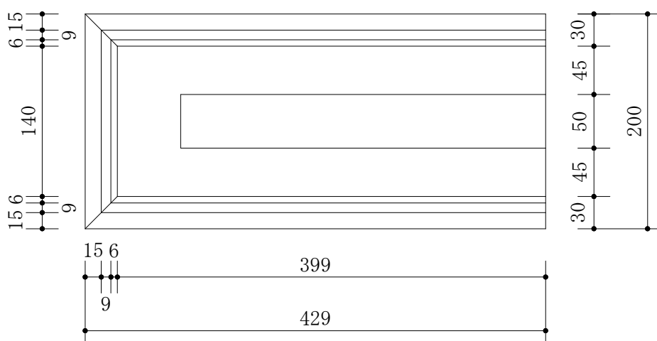
◆ 底面図
