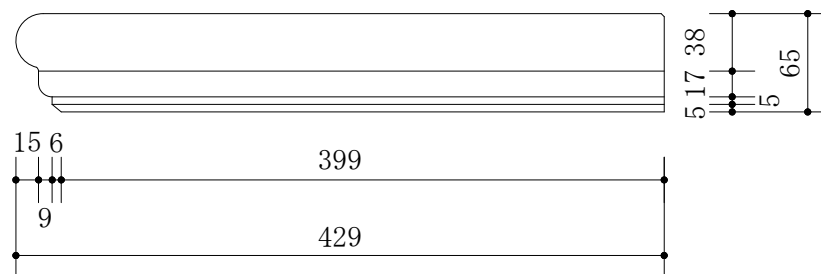
◆ 右側面図
