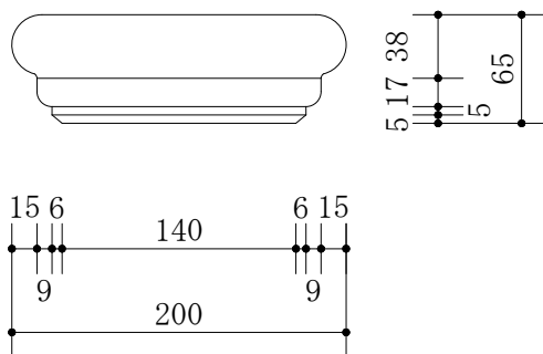
◆ 左側面図
