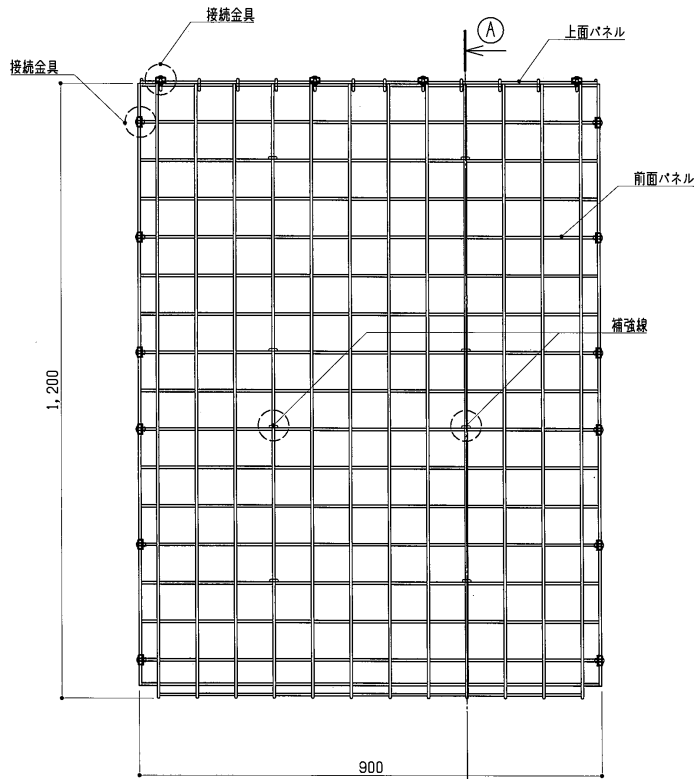
正面図 S=1:10
