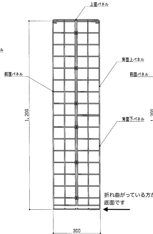
側面図 S=1:10
