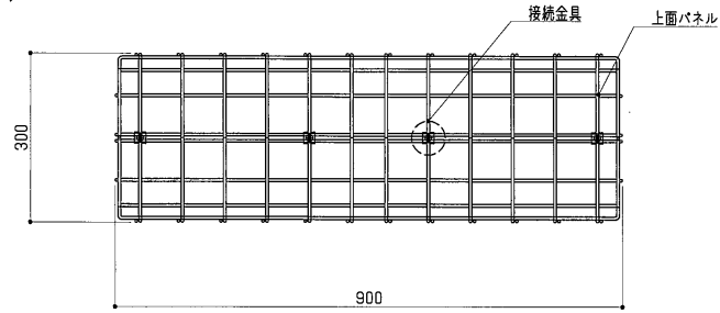
平面図 S=1:10
