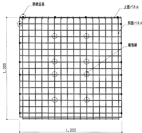
正面図 S = 1 : 15
