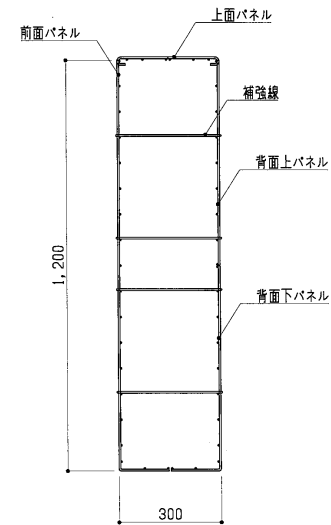
断面図 S = 1 : 15
