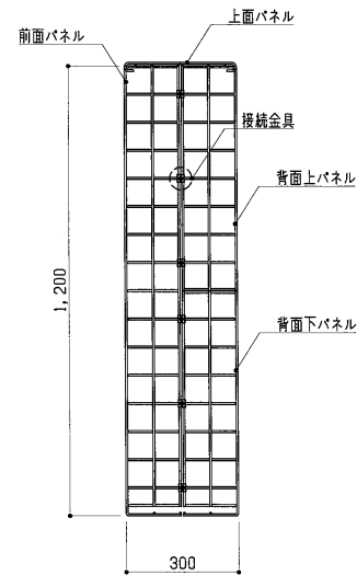
側面図 S = 1 : 15
