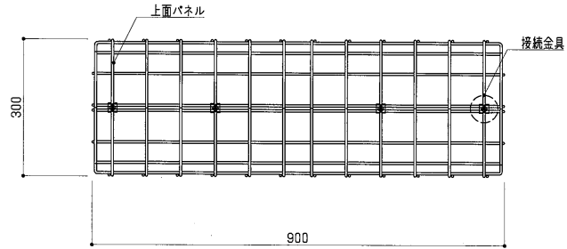
平面図 S=1:10
