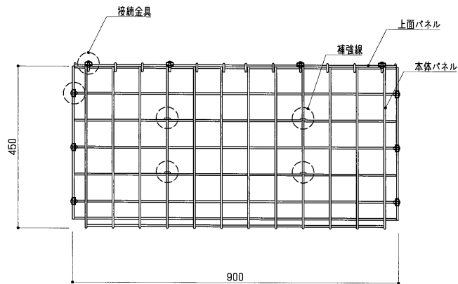
正面図 S=1:10
