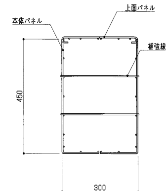
断面図 S=1:10
