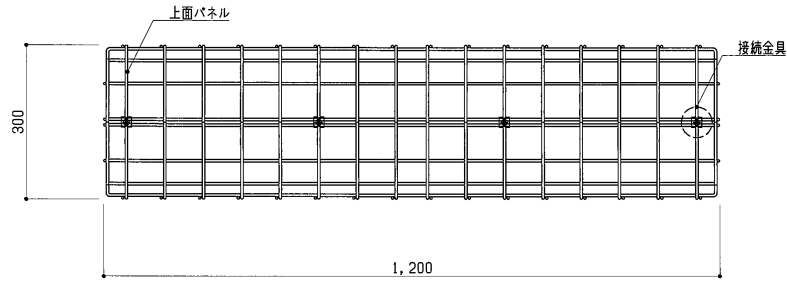
平面図 S=1:10
