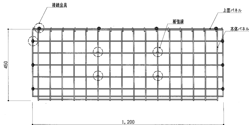
正面図 S=1:10
