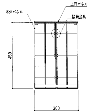
側面図 S=1:10
