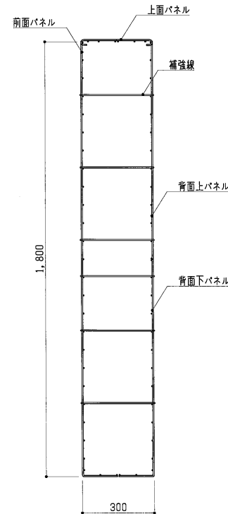
断面図 S=1:15
