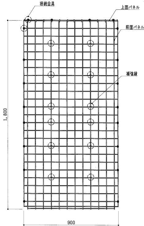
正面図 S=1:15
