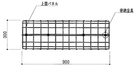
平面図 S=1:15
