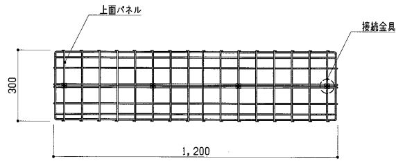
平面図 S = 1 : 15
