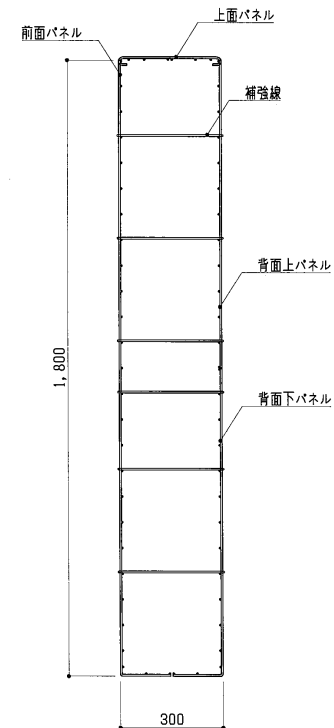
断面図 S = 1 : 15
