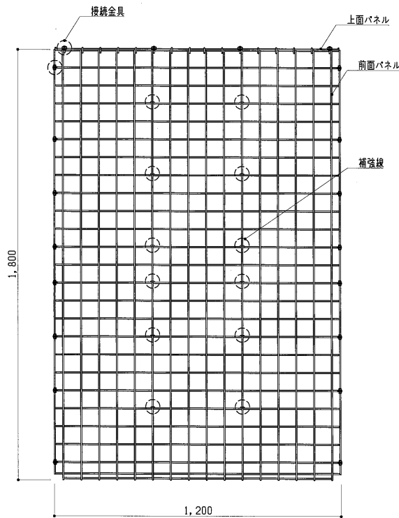
正面図 S = 1 : 15
