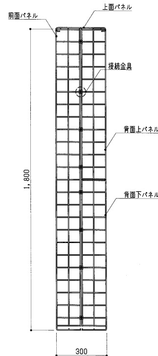
側面図 S = 1 : 15
