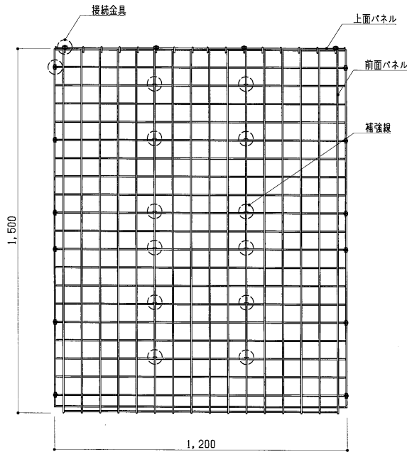
正面図 S=1:15
