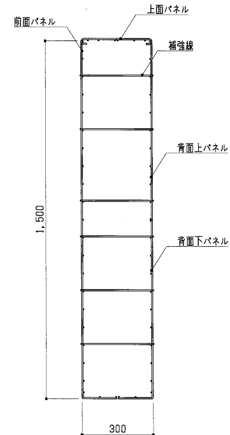
断面図 S=1:15
