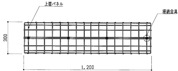
平面図 S=1:15
