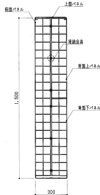
側面図 S=1:15
