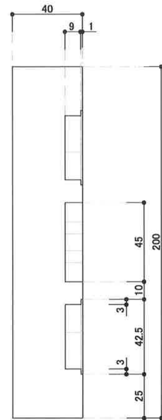
A-A'断面図S : 1/2
