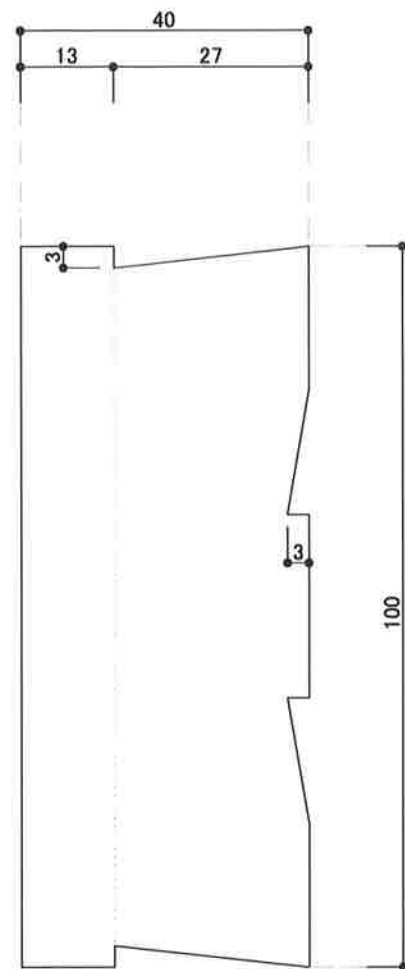
A-A`断面図S:1/1
