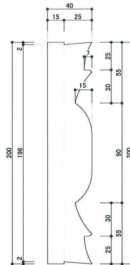
A-A'断面図S : 1/2
