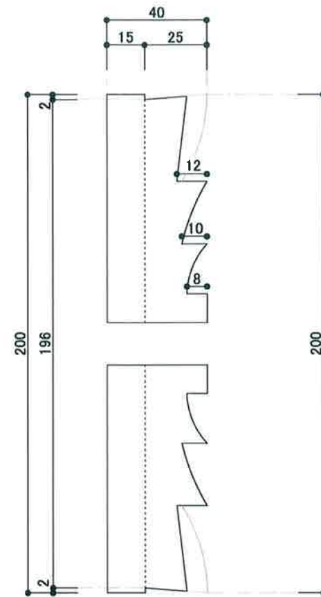
A-A' 断面図S : 1/2
